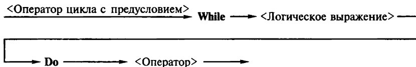
Рис. 2.16. Синтаксическая диаграмма цикла с условием
