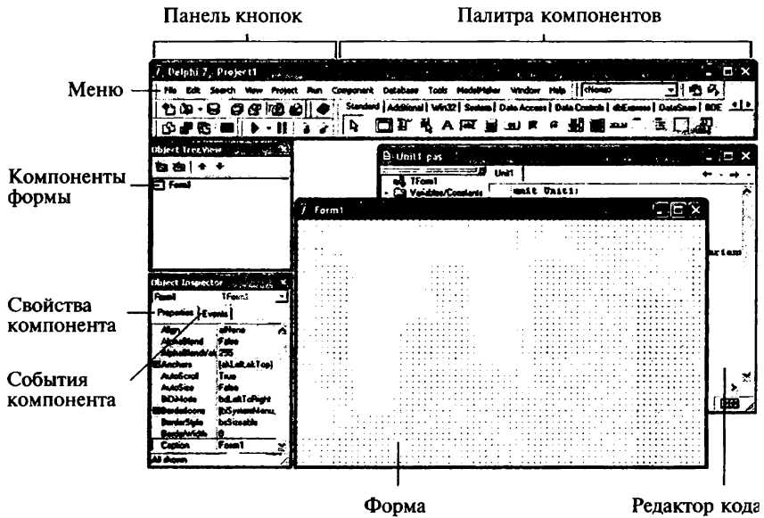
Рис. 4.2. Элементы интерфейса Delphi
