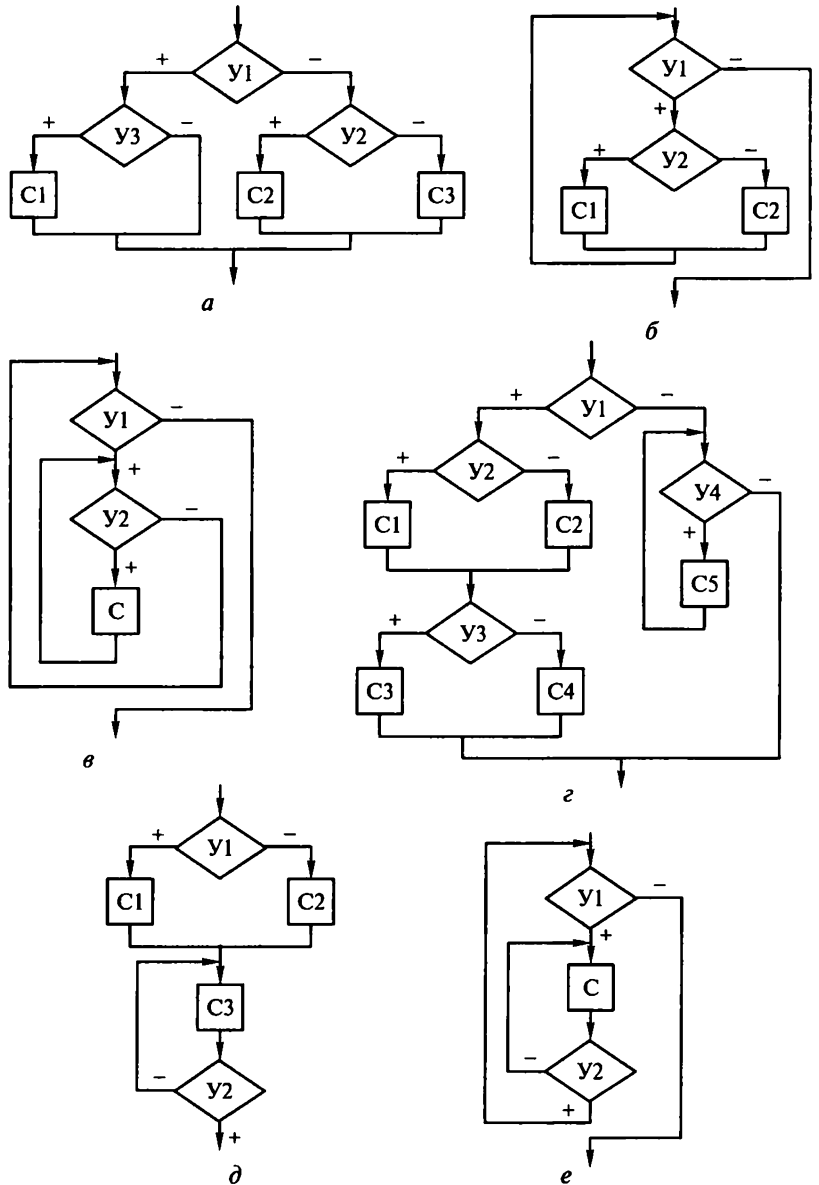
Рис. 1.13. Примеры структурных блок-схем алгоритмов:
