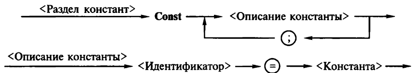
Рис. 2.4. Структура раздела констант
